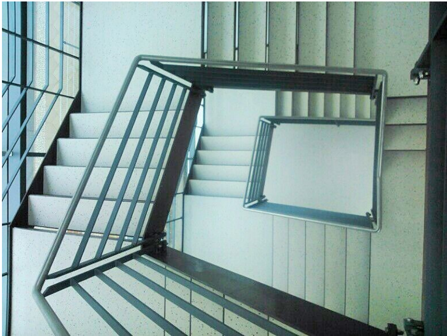
Trittstufen aus Betonwerkstein auf Treppenstahlkonstruktion
