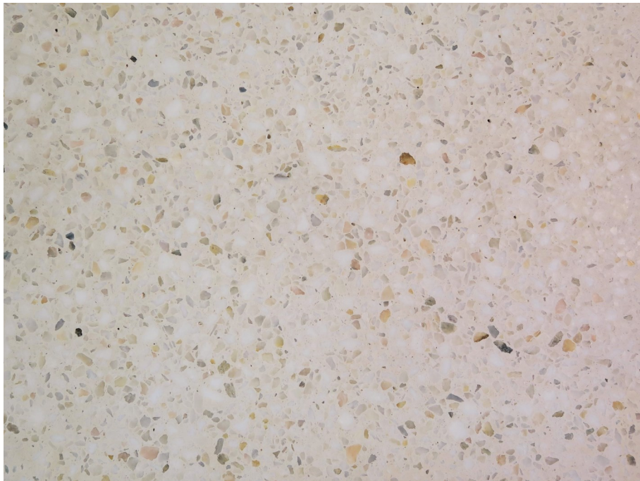
Muster CKL 1: Weiße Marmorkörnung 0-9 mm in Weißzement gebunden
